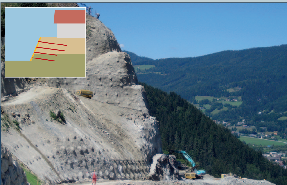
Estabilización de taludes mediante soilnailing
