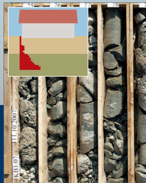
Investigación de suelos con ensayo y extracción de testigos
